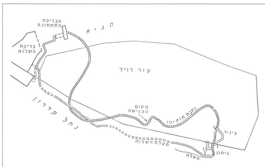
תכנית הנקבה – תעלת השילוח
